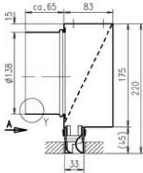
DSX-XXL S 1 Z
