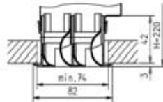
DSX-XXL P 2 Z
