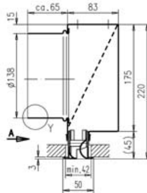
DSX-XXL P 1 Z
