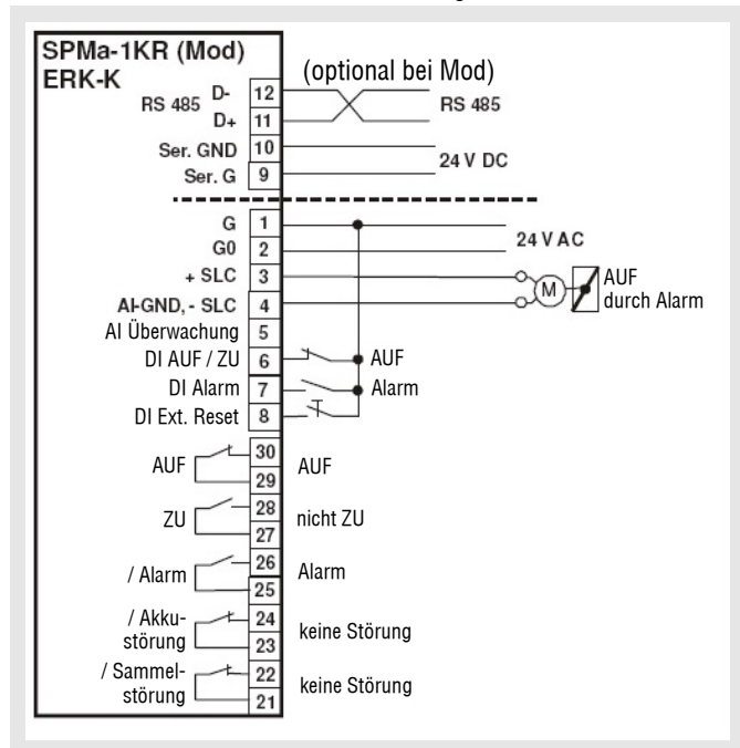
Anschlussbild Standard in Entrauchungsbetrieb
